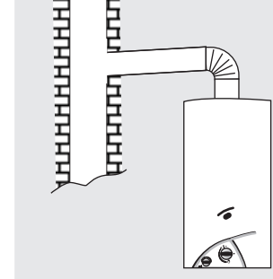
Yanlış Yatay boru eğimi aşağıya doğru verilmiş.
