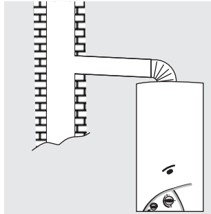
Yanlış Uzunluğu en az 33 cm olması gereken dikey boru mevcut değil.
