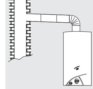
Yanlış Yataydaki boru uzunluğu 2 m'den fazla.
